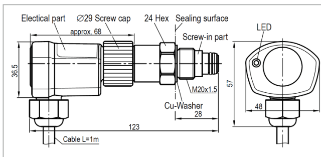
尺寸示意图
