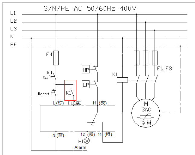
线路示意图
